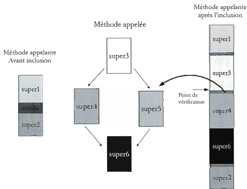
Figure 2.5 Exemple imagé d'un point de vérification
