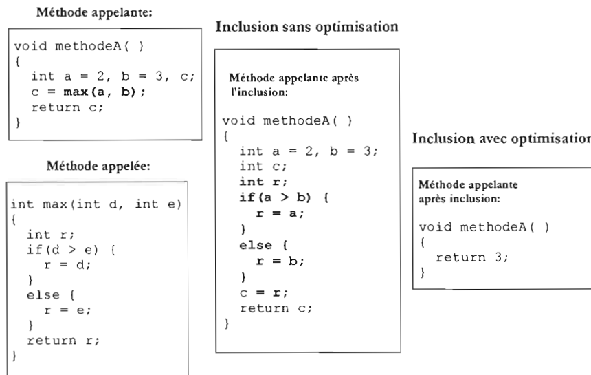
Figure 2.1 Exemple classique d'inclusion effectuée par un compilateur.
