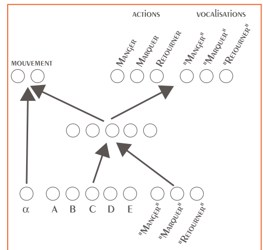
SCHEMA DE L'ARCHITECTURE DU RESEAU DE NEURONES
