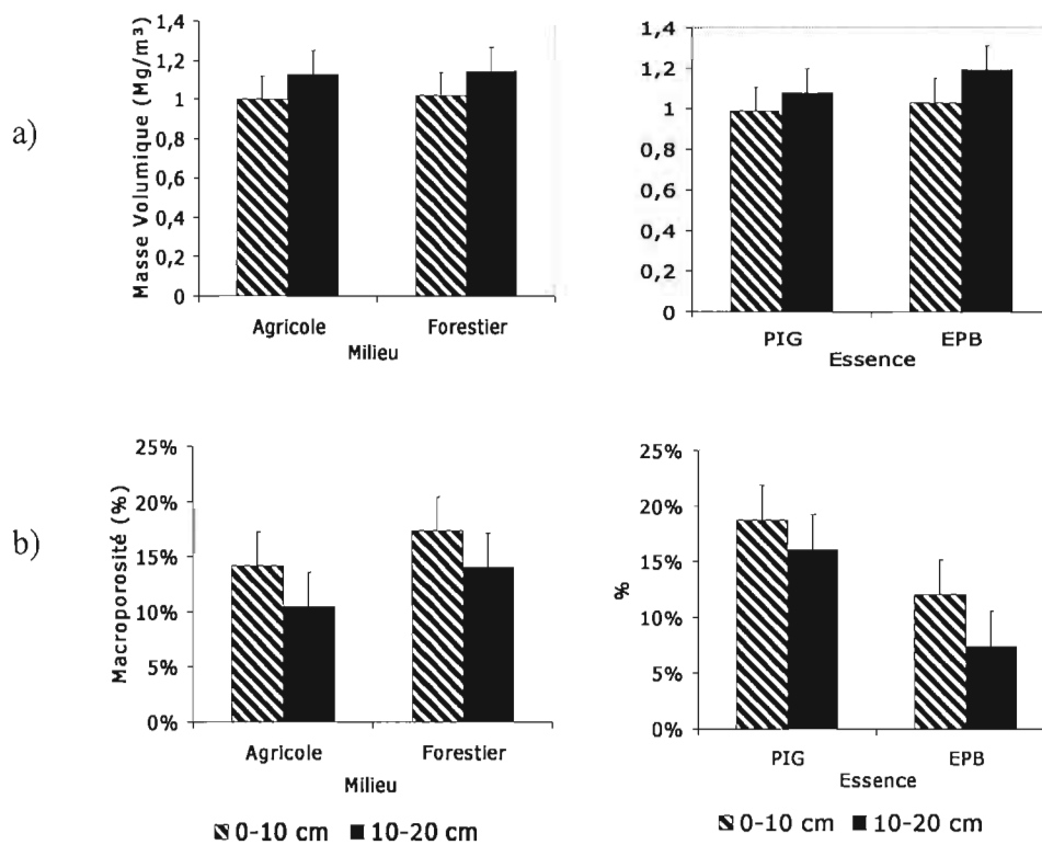
Figure 2.2 Masse volumique (a) et macroporosité (b) à 0 - 10 cm et 10 - 20 cm de profondeur en fonction des milieux et des essences. Les barres verticales représentent l'écart type de la population.
