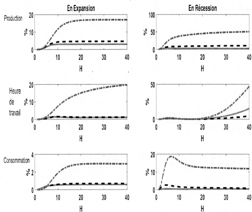
FIGURE G.1: Décomposition de variance pour le choc d'incertitude macroéconomique (cadre non linéaire)
