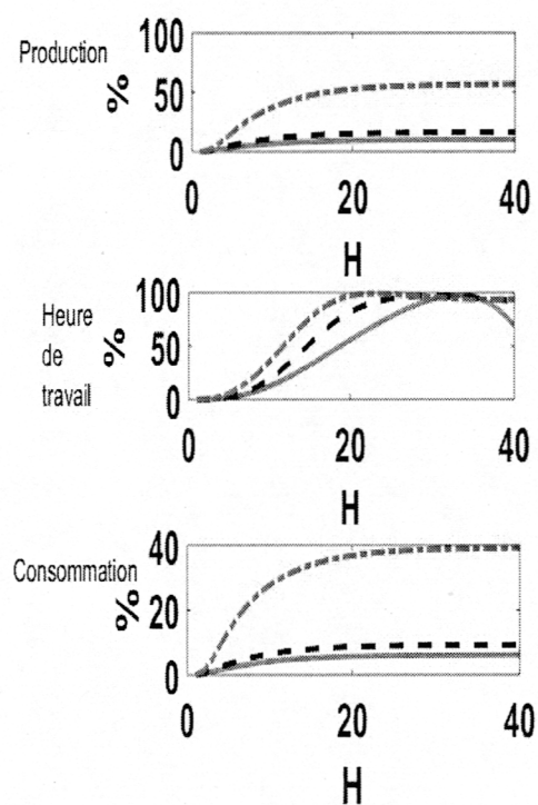
FIGURE C.1: Proportion de la variance expliquée par le choc d'incertitude macroéconomique (cadre linéaire)
