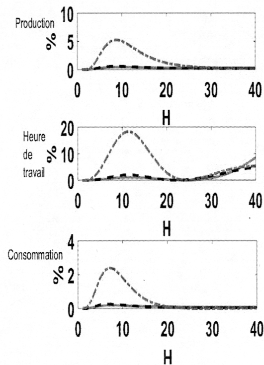
FIGURE D.1: Proportion de la variance expliquée par le choc d'incertitude financière (cadre linéaire)
