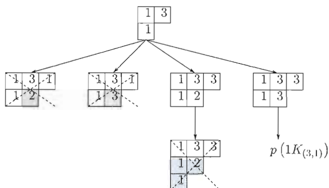
Figure 7.9 Étude du premier cas.
