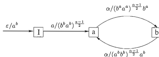
Figure 6.2 Transducteur engendrant m_{\{a,b\}} pour un alphabet impair.
