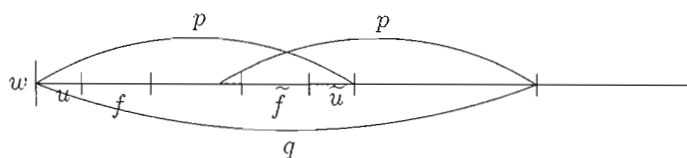
Figure 6.3 Schéma de la preuve de la Proposition 6.3.5.
