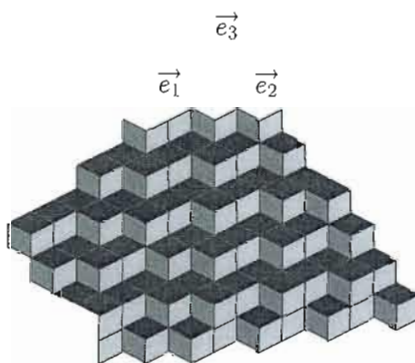
Figure 7.2 Un morceau de surface discrète.
