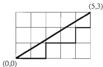
Figure 2.2 Le mot de Christoffel aabaabab de pente 3/5 .
