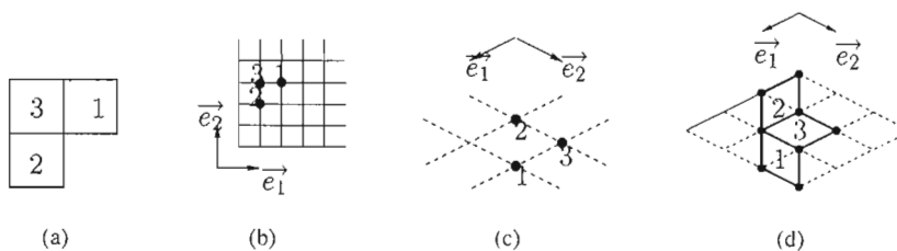
Figure 7.6 Exemple de la bijection d'un motif équerre et de sa représentation en 3 dimensions.
