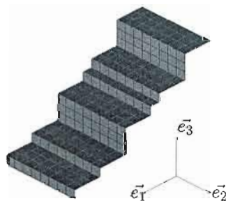
Figure 7.10 Une surface discrète associée au mot K_{(3,1)} .
