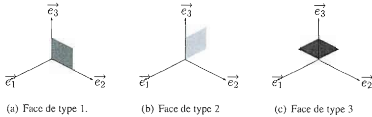
Figure 7.1 Les 3 faces fondamentales.
