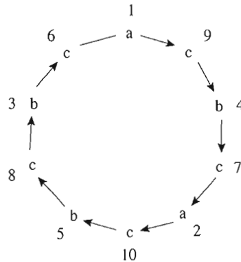
Figure 2.3 Illustration de l'Exemple 2.5.2
