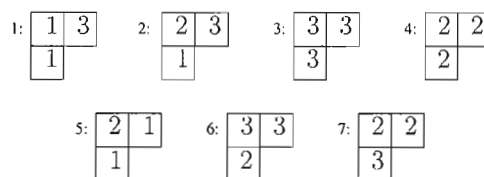
Figure 7.8 Les motifs possibles pour commencer le pavage.
