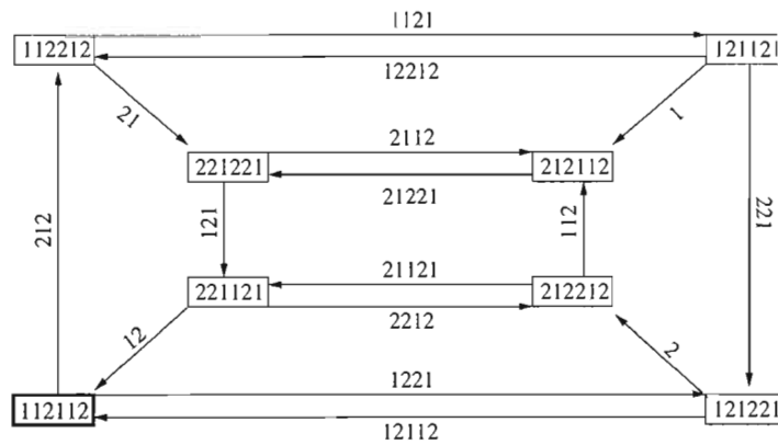
Figure 5.4 Graphe de De Bruijn d'ordre 6 réduit pour le mot m .
