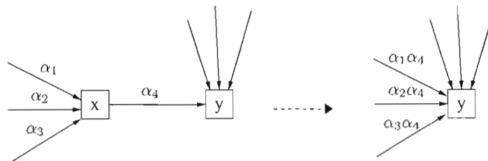
Figure 5.2 Suppression du sommet x d'un graphe de De Bruijn.
