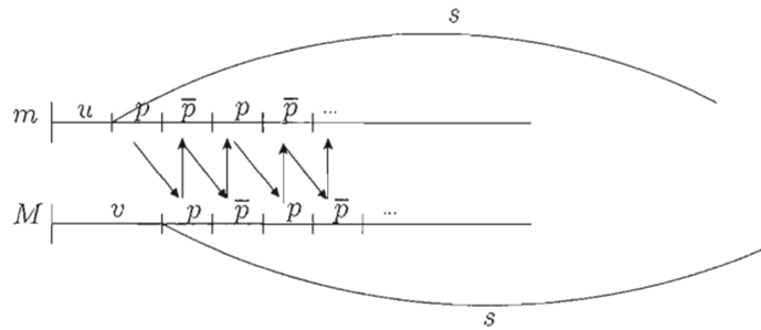
Figure 5.6 Schéma de la preuve du Lemme 5.6.5.
