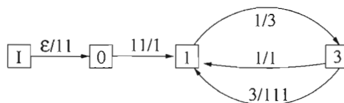
Figure 6.1 Transducteur engendrant le mot lisse minimal sur l'alphabet \{1, 3\} .
